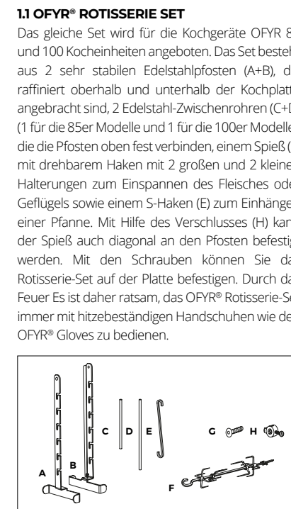
OFYR® ROTISSERIE SET - TEILE
