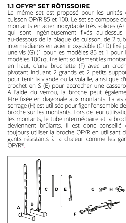
OFYR® SET RÔTISSOIRE - PIÈCES
